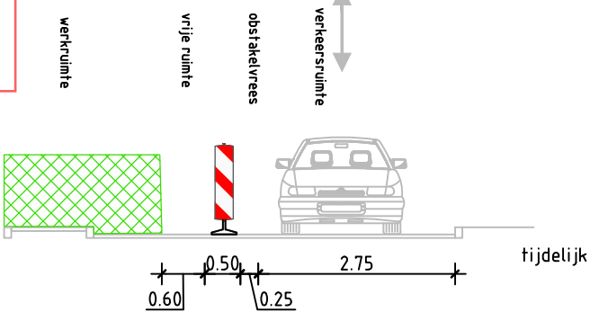
Dwarsprofiel A-A
