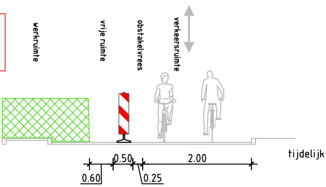
Dwarsprofiel A-A
