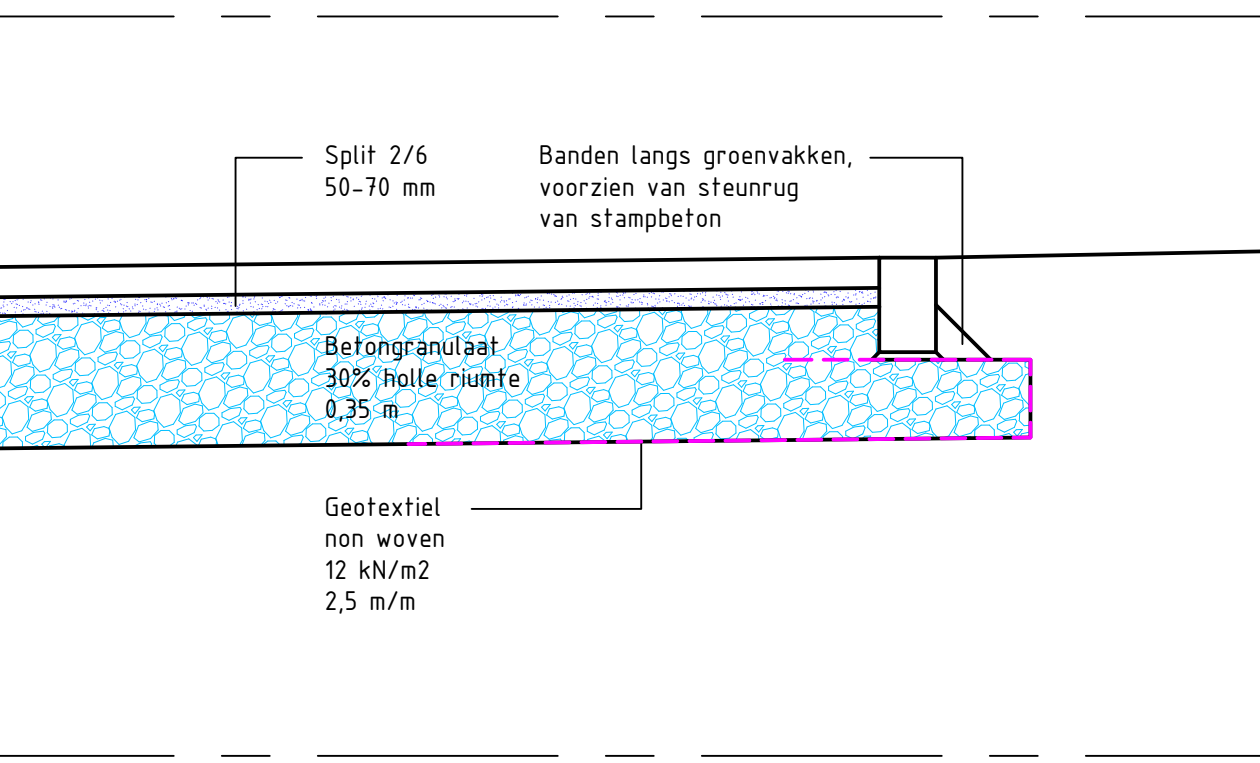
Principedetail inspakken fundering met geotextiel 1:20
