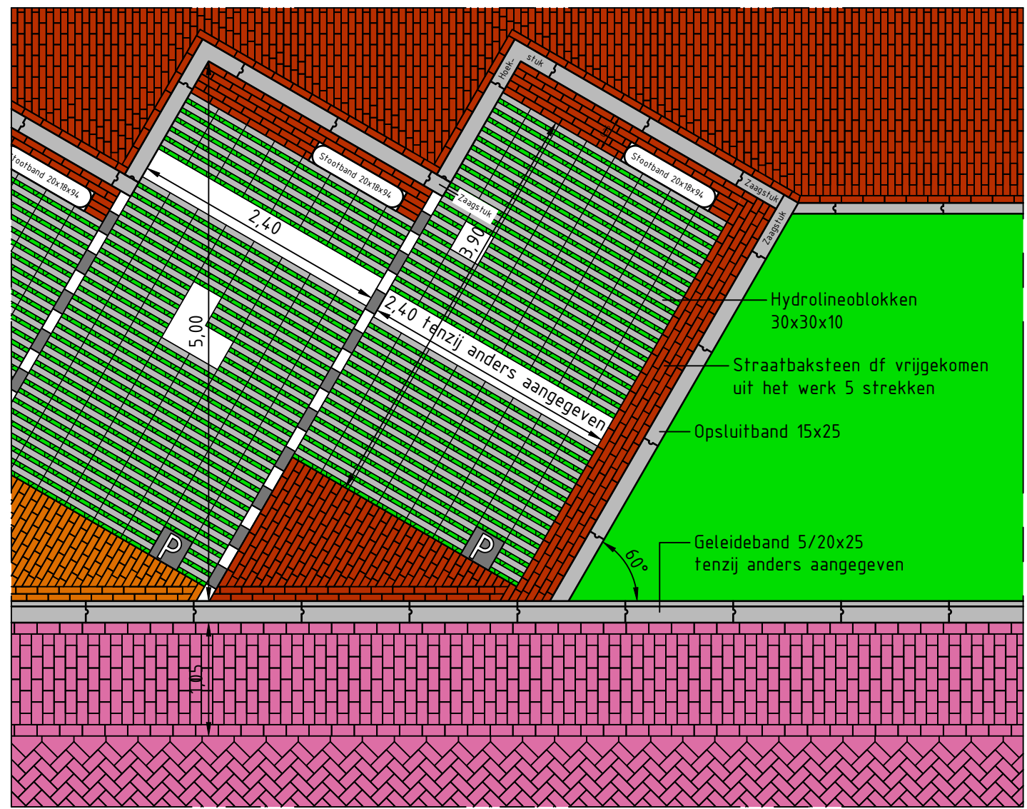
Principedetail schuin parkeren 1:50
