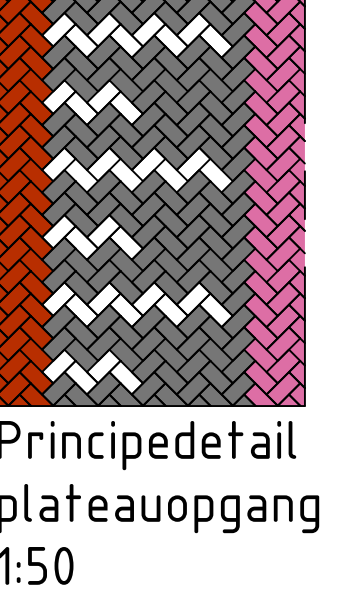
Principedetail plateauopgang 1:50
